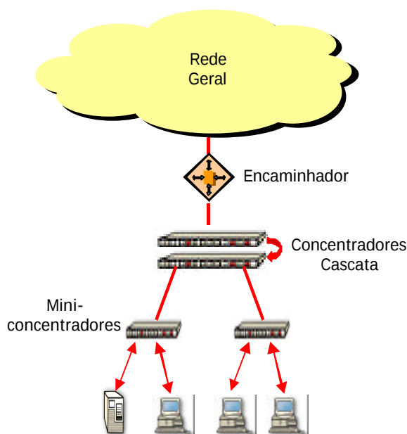
Figura 5.31 – Configuração interna da rede do CEFASI.
